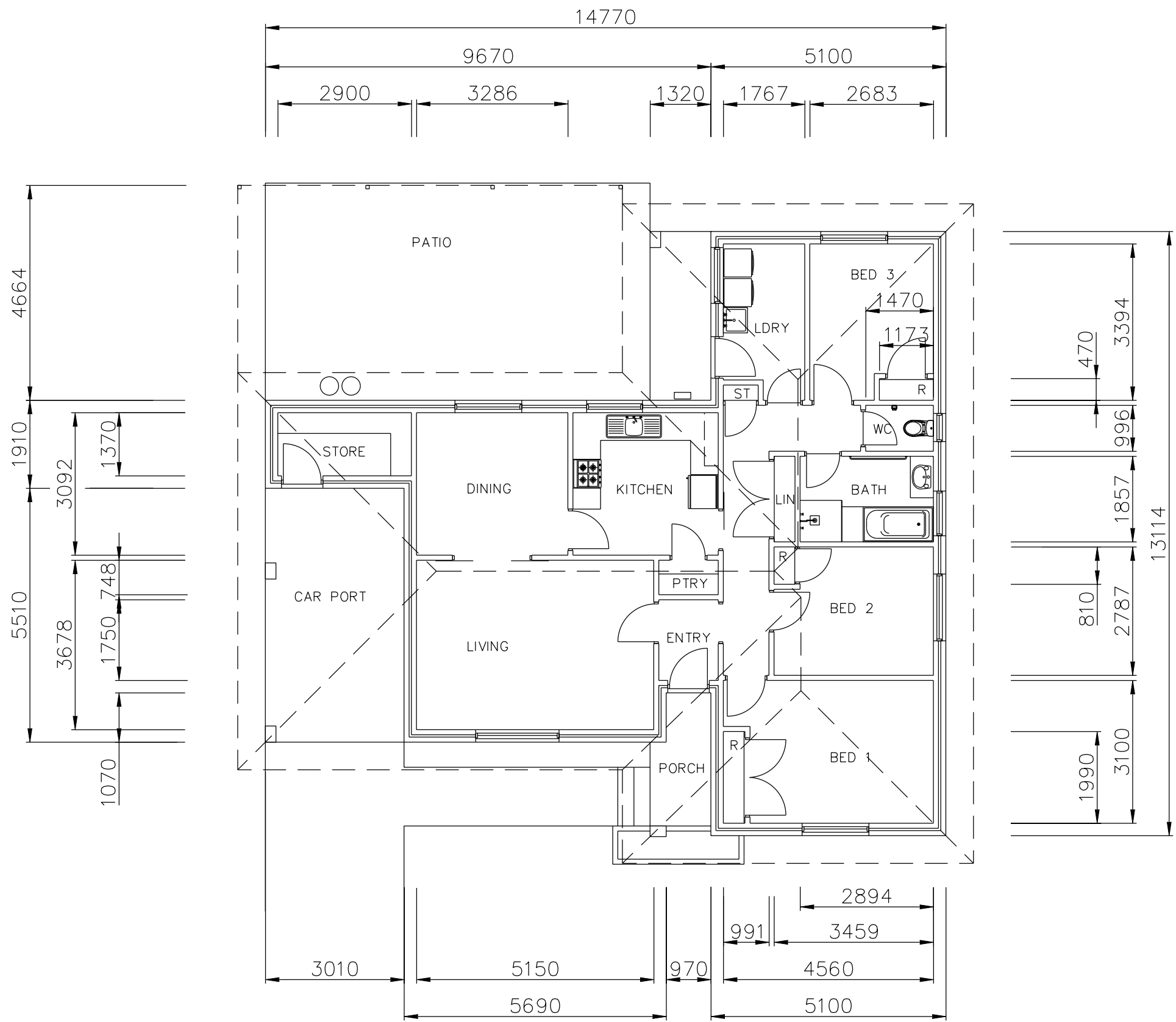
FLOOR PLAN 1 : 100
